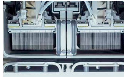
2017 Stapelfaservernadelungsline
